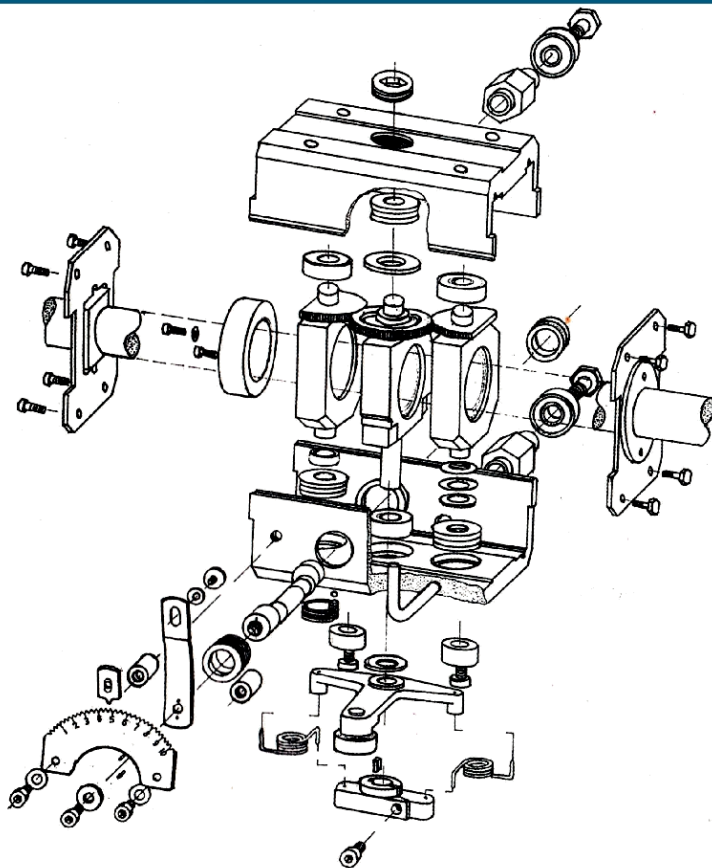
光杆排线器主机的形象以拆卸的形式出现
